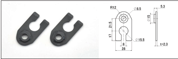
●ホースクランプステー SWCL4-ST2(21.5)
