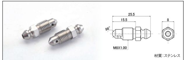
●ブリーダプラグ M8×P1.00 L15.5
