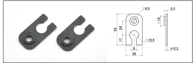
●ホースクランプステー SWCL4-ST(24)
