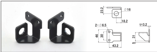
●ホースクランプステー ST205A-1RL
