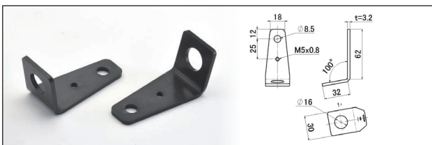
●ホースクランプステー FD2
