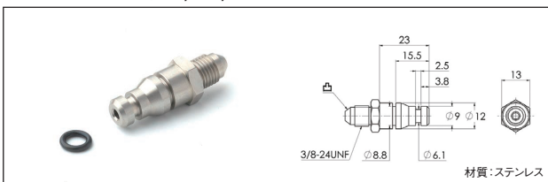
●クラッチラインアダプター φ12-φ9 15.5 - AN3
