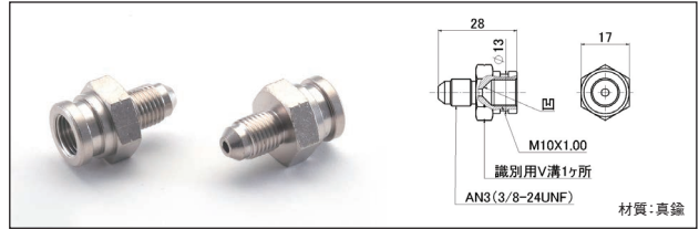
●フレアナットアダプター M10×P1.00IF メス凹 - AN3
