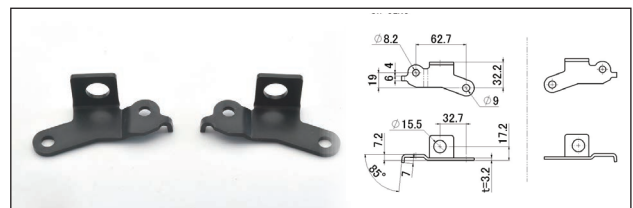
●ホースクランプステー NCEC-RL
