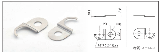
●ホースクランプステー CV5W-RL
