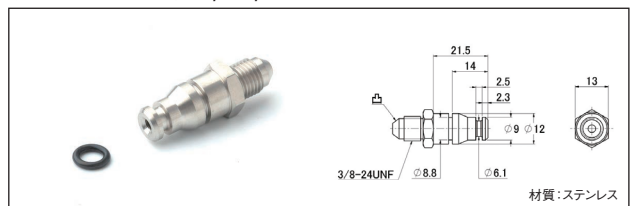
●クラッチラインアダプター φ12-φ9 14.0 - AN3
