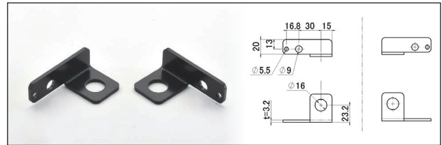
●ホースクランプステー ST205-2RL
