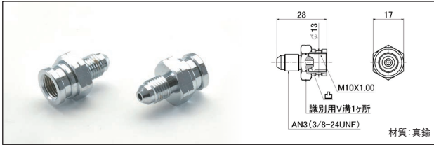
●フレアナットアダプター M10×P1.00IF メス凸 - AN3
