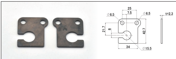
●ホースクランプステー AP2
