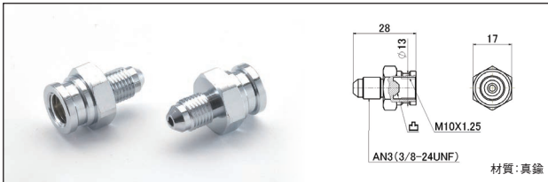
●フレアナットアダプター M10×P1.25IF メス凸 - AN3
