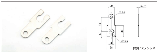
●ホースクランプステー SWCL4-ST3(45)
